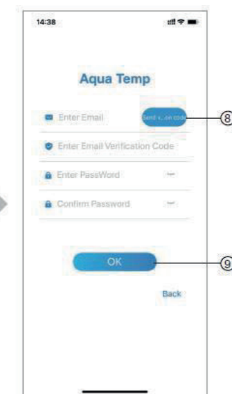
Abb. 3 Passwort vergessen-Oberfläche
