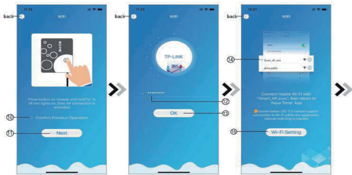
Abb. 7 WIFI-Modul AN-Oberfl.
