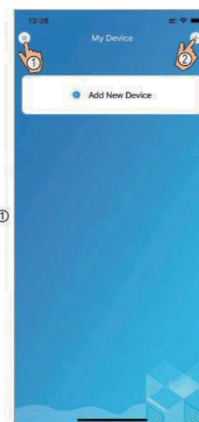
Rys. 4 Moje urządzenie
