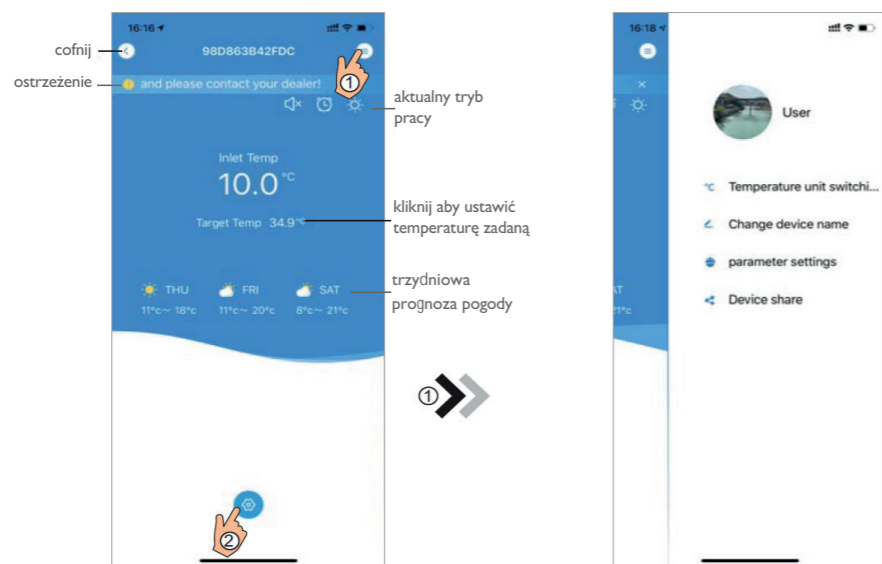
Rys. 18 Menu główne
