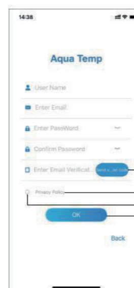
Fig. 2 Kontotilmeldings-grænseflade
