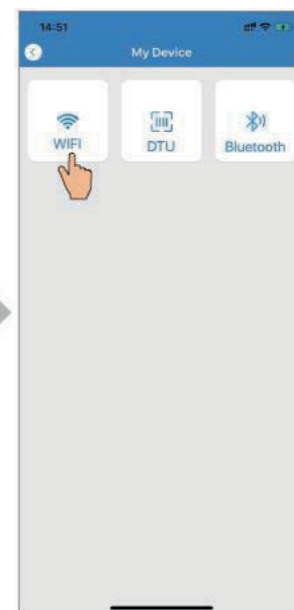
Abb. 6 Gerät hinzufügen-Oberfl.
