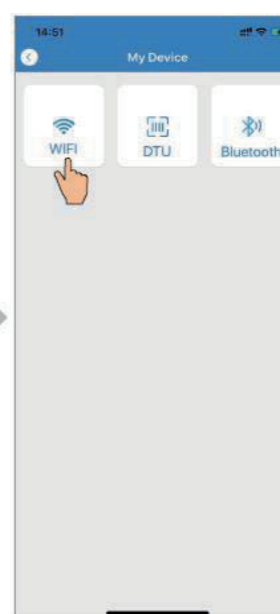
Fig. 6 Toestel toevoegen
