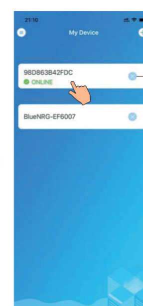
Fig. 17 Grænsefladen Enhedsadministration
