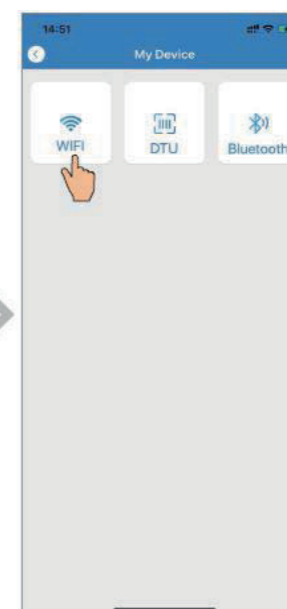
Fig. 6 Grænsefladen Tilføj
