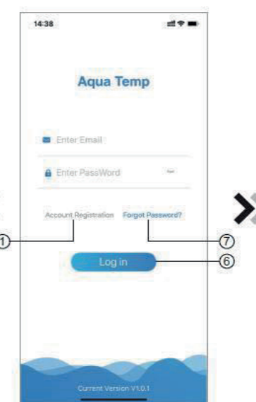
Fig. 1 Login interface
